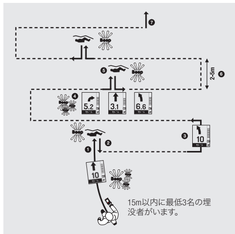
代替サーチモードでの接近している複数埋没者の捜索戦術
